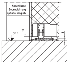
Schwellesser Bodenabschluss für einbruchhemmende Türen mit Panikfunktion
