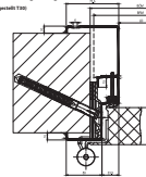
Eck- und Gegenzarge Einwegwerk Tisch
