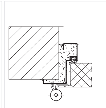
MIT MÖRTEL
