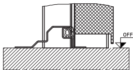
Schwelle RS bzw. BA6
