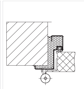
MIT BRANDSCHUTZSCHAUM
