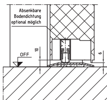
Schwellerloser Bodenabschluss für einbruchhemmende Türen mit Panikfunktion
