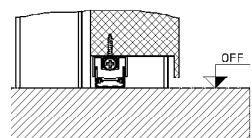
absenkbarer Bodendichtung (optional Rauchschutz)
