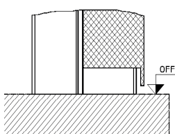
Ohne Bodeneinstand (Standard)
