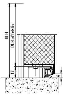
Schwelle BA1 (kein Rauchschutz)
