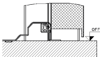
Schwelle BA 6 (optional Rauchschutz)
