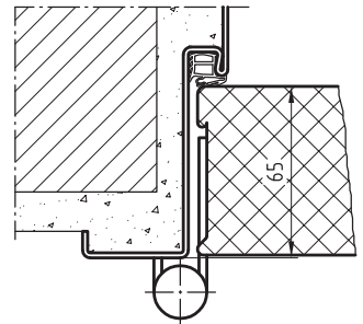
stumpfes Türblatt
