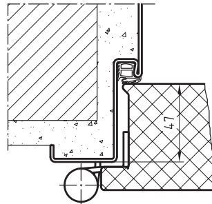
gefälztes Türblatt
