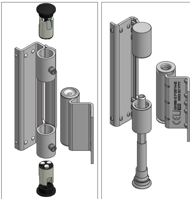
Bandsystem Variante 1
