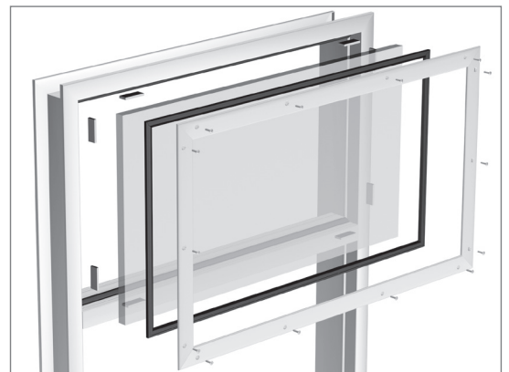
Glasleistensystem P14
