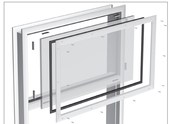
Glasleistensystem P15
