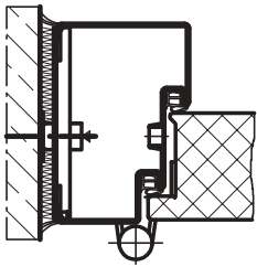
Profil 86_D BRMB = DLB + 180 BRMH = DLH + 90
