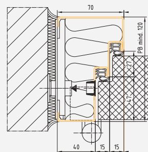
Profil 79D BRMB = DLB + 160 mm BRMH = DLH + 80 mm
