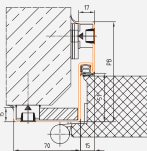
Profil 88_D BRMB = DLB + 50 mm BRMH = DLH + 25 mm
