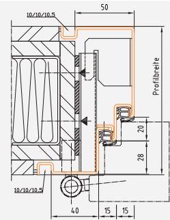
Profil 178_G
