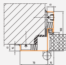
Profil 23_D BRMB = DLB + 50 mm BRMH = DLH + 25 mm
