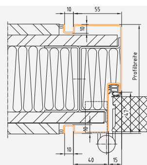
Profil 45_G
