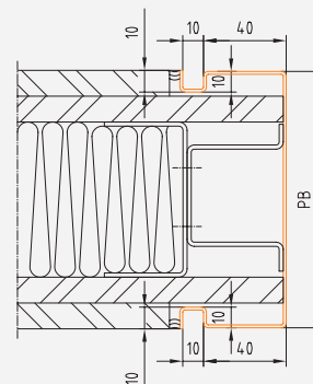
Profil 36_G
