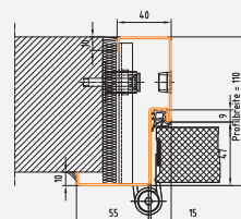
Profil 205 BRMB = DLB + 100 mm BRMH = DLH + 50 mm
