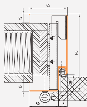
Profil 101 G
