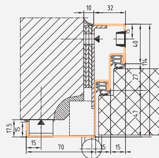
Profil 183 BRMB = DLB + 84 mm BRMH = DLH + 42 mm
