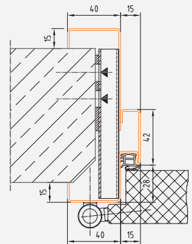
Profil 102_D2
