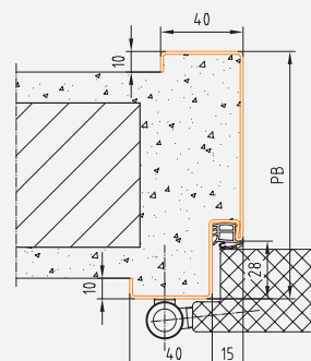
Profil 42_M
