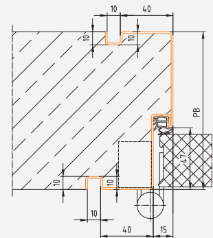
Profil 47_S
