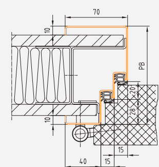
Profil 80_G
