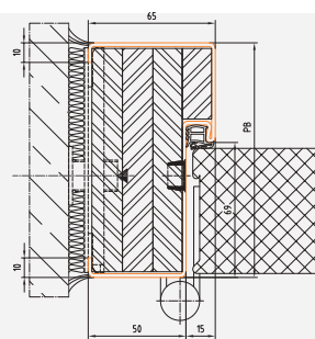
Profil 96_D
