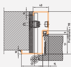
Profil 206 BRMB = DLB + 100 mm BRMH = DLH + 50 mm
