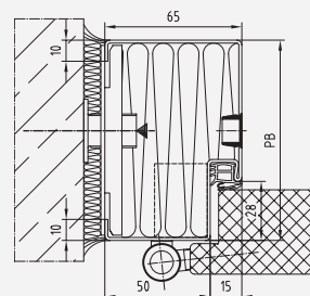
Profil 56 D
