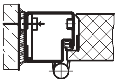
Profil 85_D BRMB = DLB + 150 mm BRMH = DLH + 75 mm
