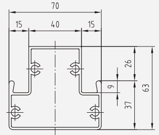
Kämpferprofil 992
