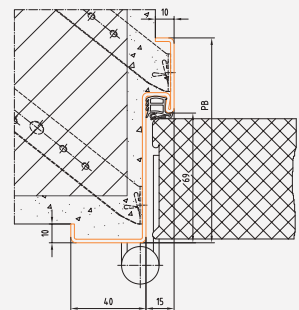
Profil 01_M
