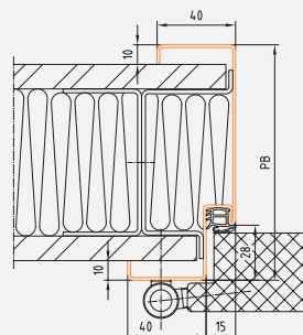
Profil 42 G
