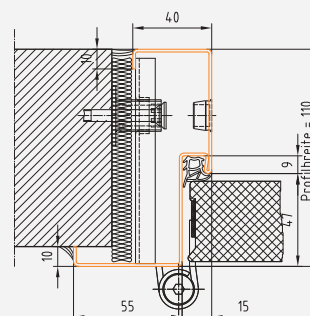
Profil 205 BRMB = DLB + 100 mm BRMH = DLH + 50 mm
