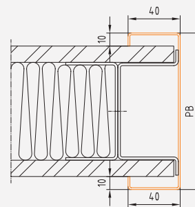
Profil 05_G BRMB = DLB + 96 mm BRMH = DLH + 48 mm
