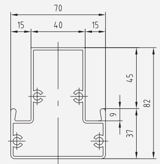
Kämpferprofil 991
