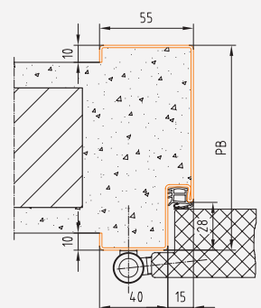
Profil 44_M BRMB = DLB + 130 mm BRMH = DLH + 65 mm
