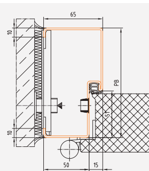
Profil 89_D BRMB = DLB + 150 mm BRMH = DLH + 75 mm
