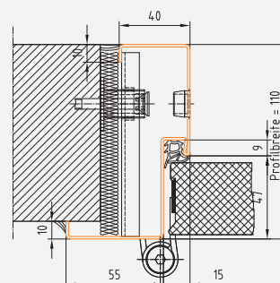
Profil 205
