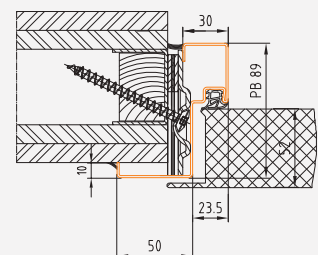
Profil 377
