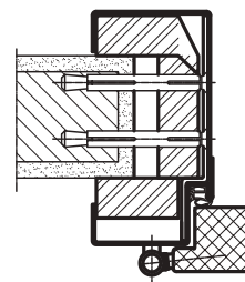
PROFIL 66 Seite 32
