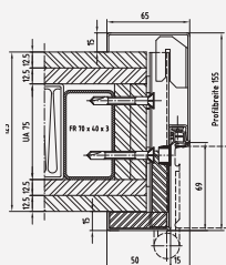
Profil 164_G
