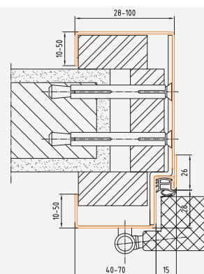
Profil 66
