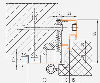
Profil 184 BRMB = DLB + 84 mm BRMH = DLH + 42 mm
