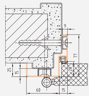
ZARGEN
