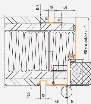
Profil 47_G
