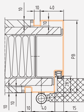
Profil 48_G
