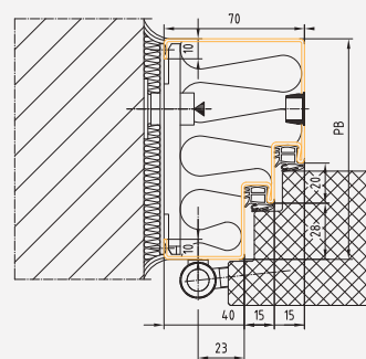
Profil 80D BRMB = DLB + 160 mm BRMH = DLH + 80 mm
