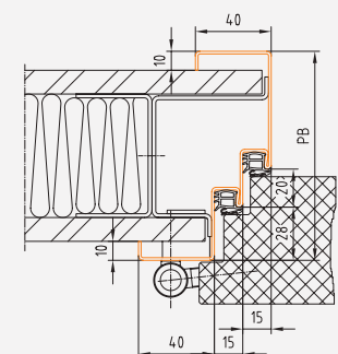
Profil 82_G
