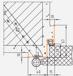
Profil 22_M
