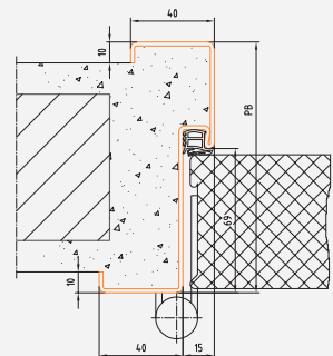
Profil 15_M
