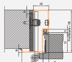
Profil 206 BRMB = DLB + 100 mm BRMH = DLH + 50 mm
