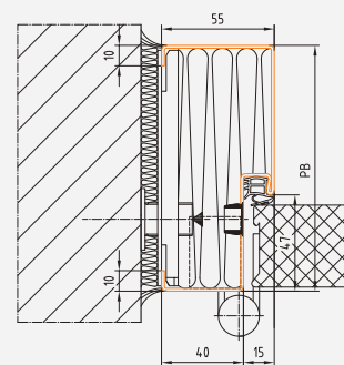
Profil 43_D BRMB = DLB + 130 mm BRMH = DLH + 65 mm
