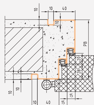
Profil 38_M BRMB = DLB + 120 mm BRMH = DLH + 60 mm
