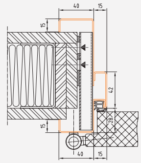
Profil 102_G
