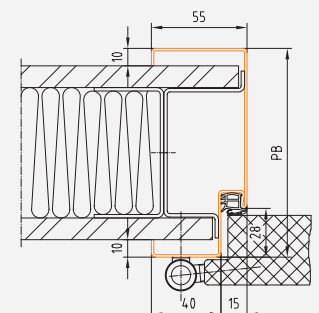
Profil 44_G
