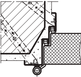
Mauermontage M
