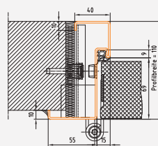
Profil 207 BRMB = DLB + 100 mm BRMH = DLH + 50 mm
