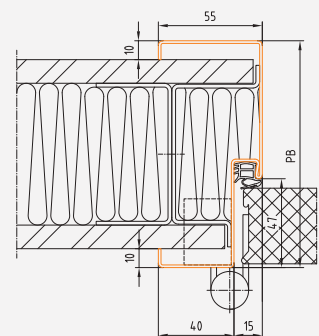
Profil 43_G
