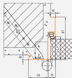
Profil 21_M BRMB = DLB + 50 mm BRMH = DLH + 25 mm
