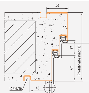
Profil 37_S
