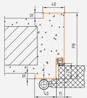
Profil 42_M BRMB = DLB + 100 mm BRMH = DLH + 50 mm
