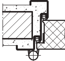
Profil 513_MM
