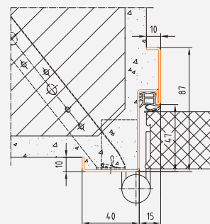
Profil 21 M
