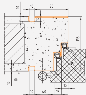
Profil 78_M BRMB = DLB + 180 mm BRMH = DLH + 90 mm
