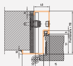
Profil 206 BRMB = DLB + 100 mm BRMH = DLH + 50 mm
