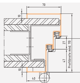
Profil 79_G
