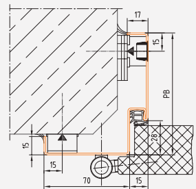
Profil 24_D
