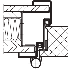
Profil 513_G (für UT60x) BRMB = DLB + 127 mm BRMH = DLH + 63 mm
