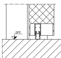
Schwelle BA1 (optional Zeitverzögert)
