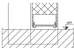
Schwelle BA1 (0-220 mm auf Wunsch möglich)
