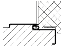
Türblatt 4-seitig gefälzt Zarge 4-seitig umlaufend
