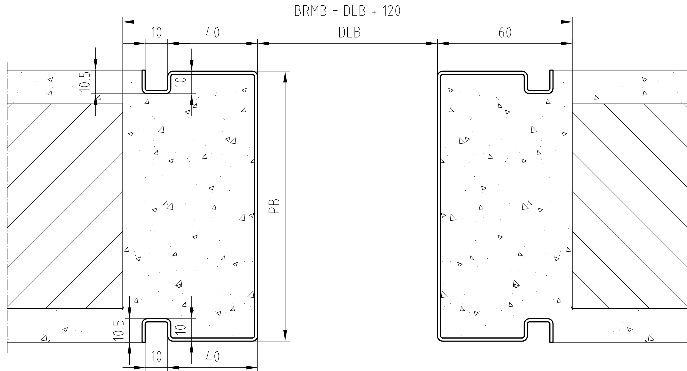
D_Durchgangszarge_36_M.dwg
