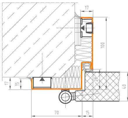
OBEJMUJĄCA DWUCZĘŚCIOWA P101
