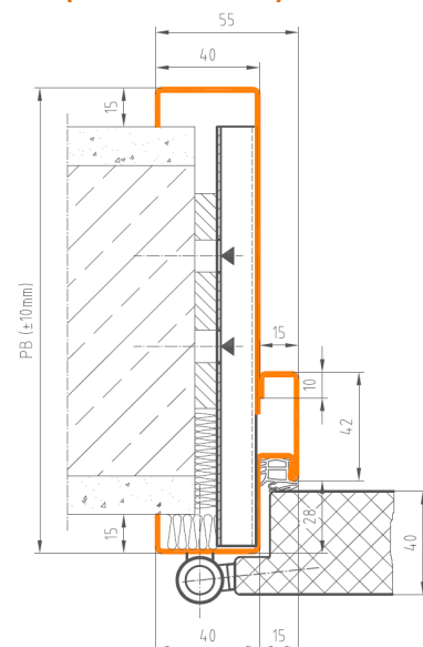
OBEJMUJĄCA DWUCZĘŚCIOWA P103 (REGULOWANA)
