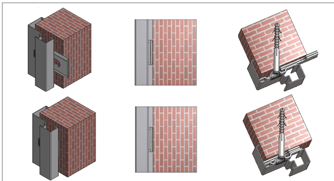
Abb.10.1 Positionierung der Stahlblechdistanzen
