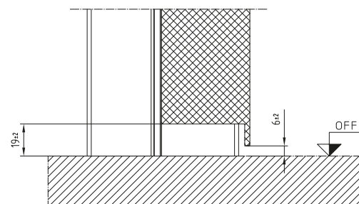
Abb. 17.1.1: unterer Türblattabschluss, 3-seitig
