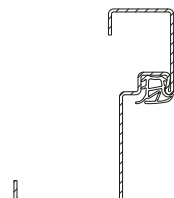
Abb. 14.2: Dichtung C560 für Zargenprofil 25, 26, 53 und 377
