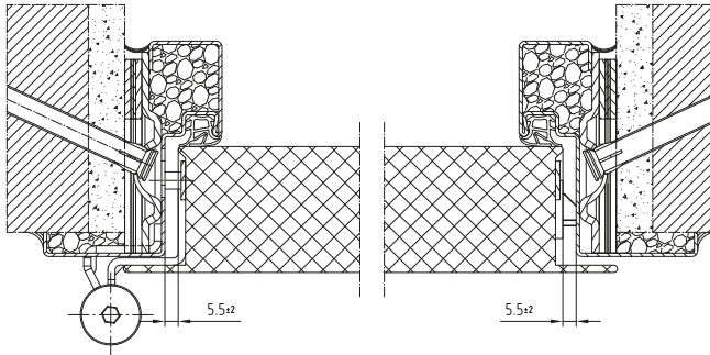
Abb. 17.1.2: Band- und Schlossseite
